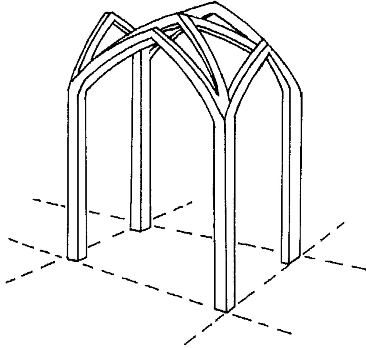
شكل (١١) عقد مدبب، مضلع مصلب
